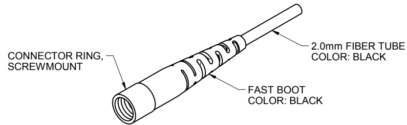
2.0mm FXC-series BOOT
